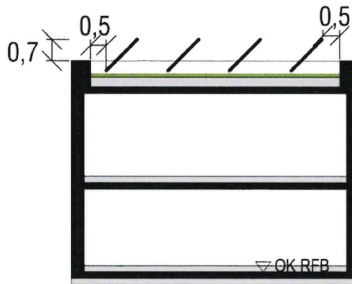
Schematische Abbildungen zur Höhe der Module bei Solarenergienutzung (mit beispielhafter Aufständerung)
